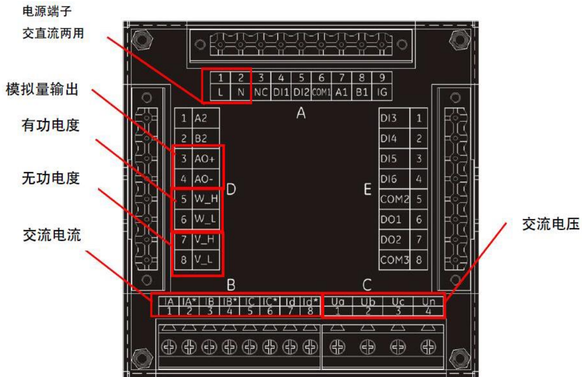
图 3.3 DH-MFMS-1V01 背部端子图
