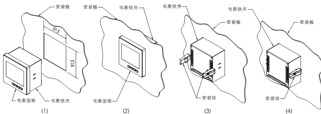
图 3.1 智能三相多功能电力仪表安装图
